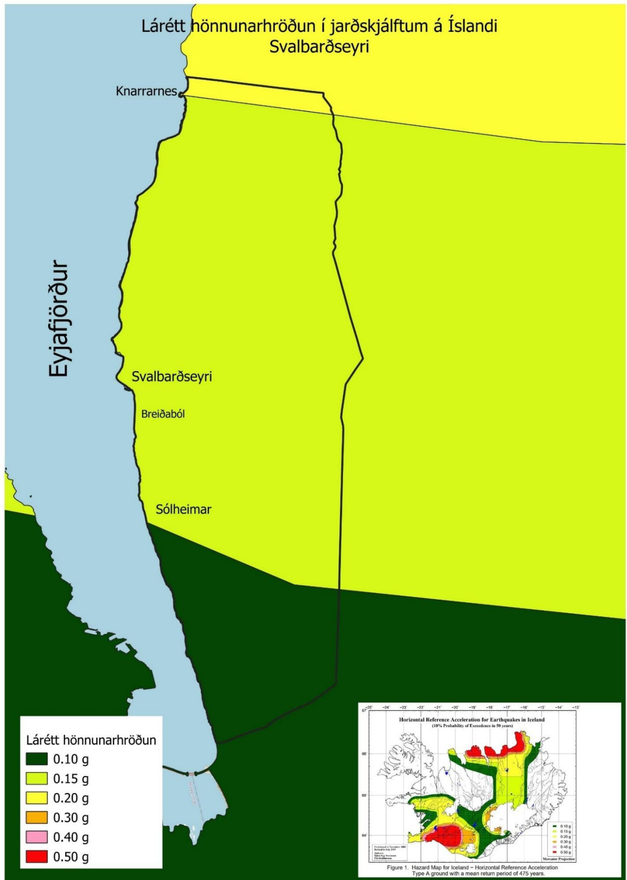
Mynd 39 Áætlun um hönnunarhröðun eftir svæðum í Svalbarðsstrandarhreppi
